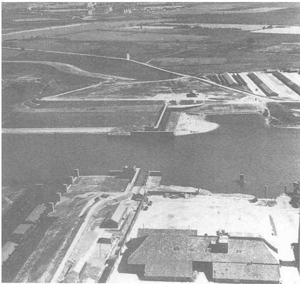
2.3. De stuw in de Nederrijn. (Herkomst: DS)
