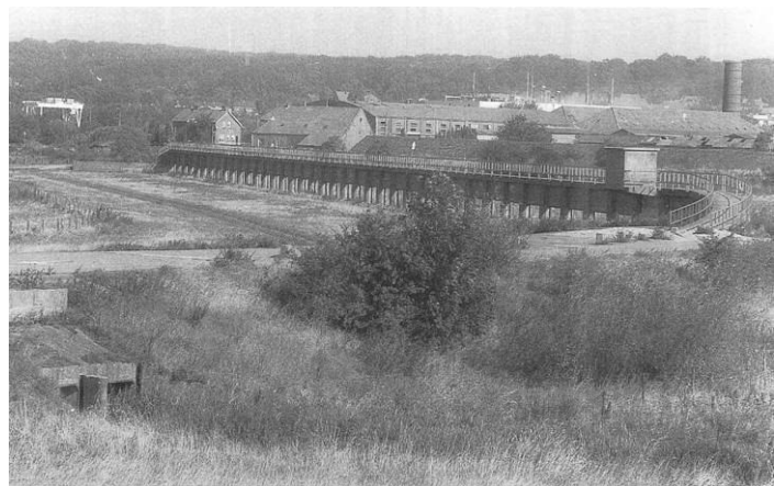
2.7. Militaire doorlaatbrug met overlaatl dijken en sluisje in de polder Meinerswijk, omstreeks 1960. (Herkomst: YL.)
